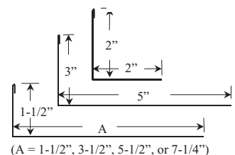
22. Angle Trim
