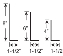
21. 4", 6", & 8" Fascia Trim
