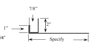
18. Overhead Door Trim
